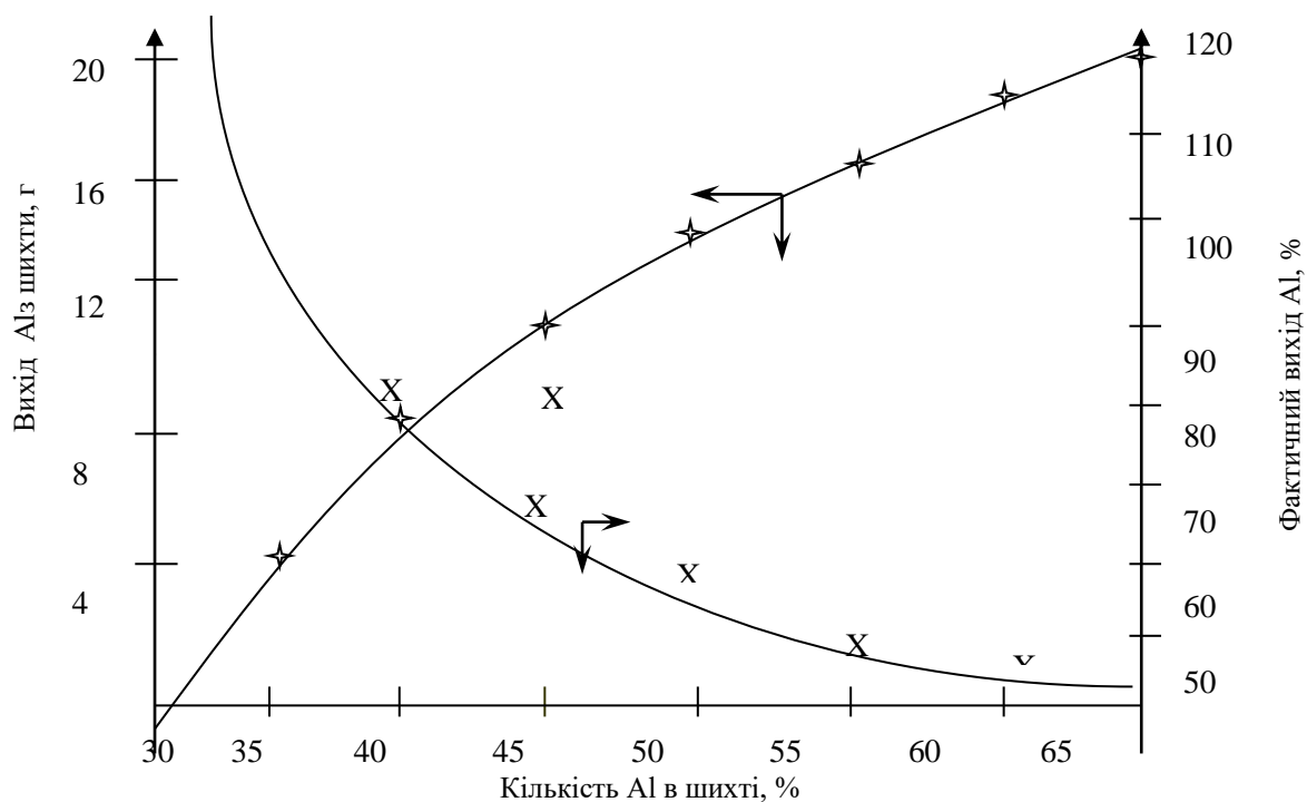
Рис. 1. Графічна залежність виходу Al з шихти: - вихід металу, г; X - фактичний вихід металу у порівнянні з розрахованим, %
